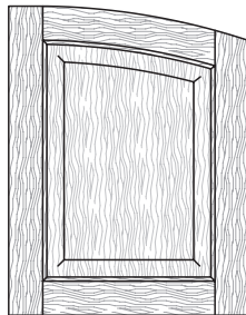
Style: 2011R PC: 123 Frame: PC123 x 0.6 Min. Size: 8x9¼
